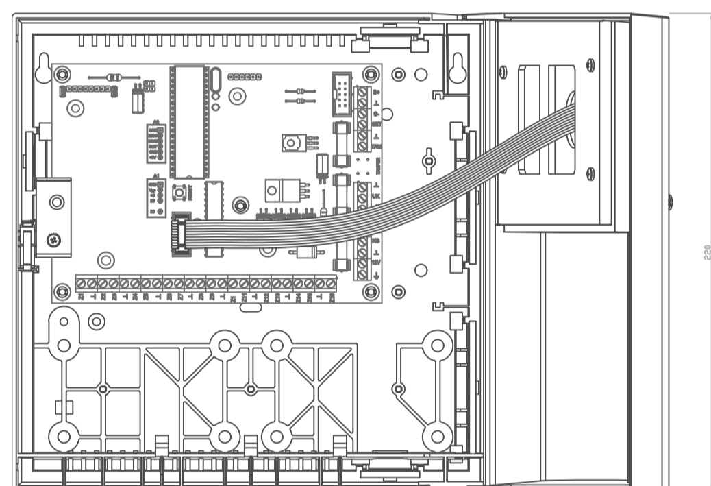
ПККОП "Данна-16/32" (крышка открыта)
