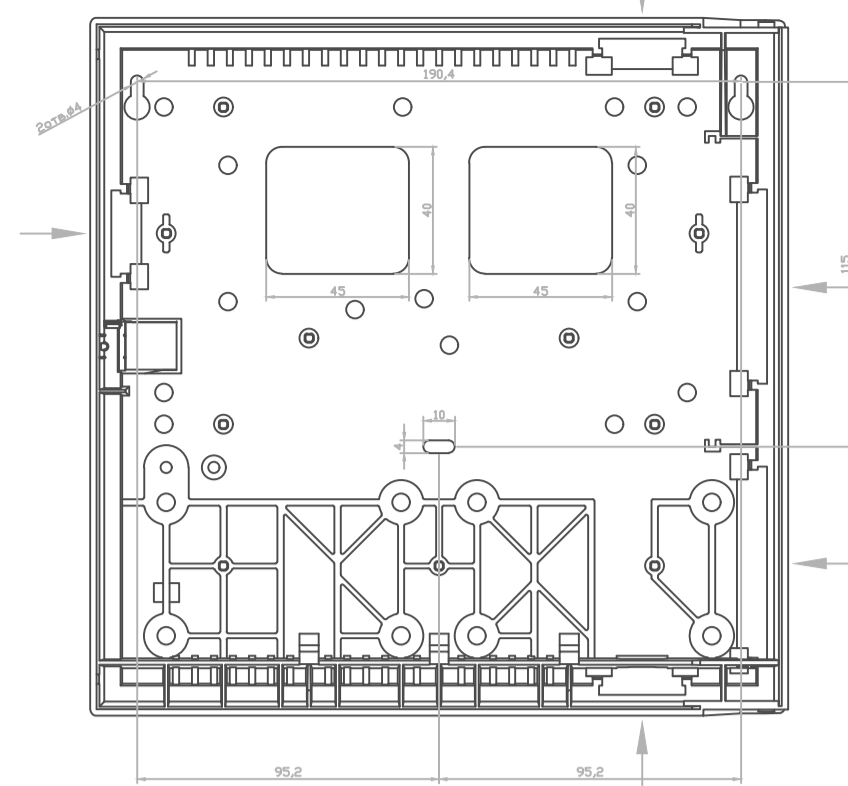
Монтажные отверстия
