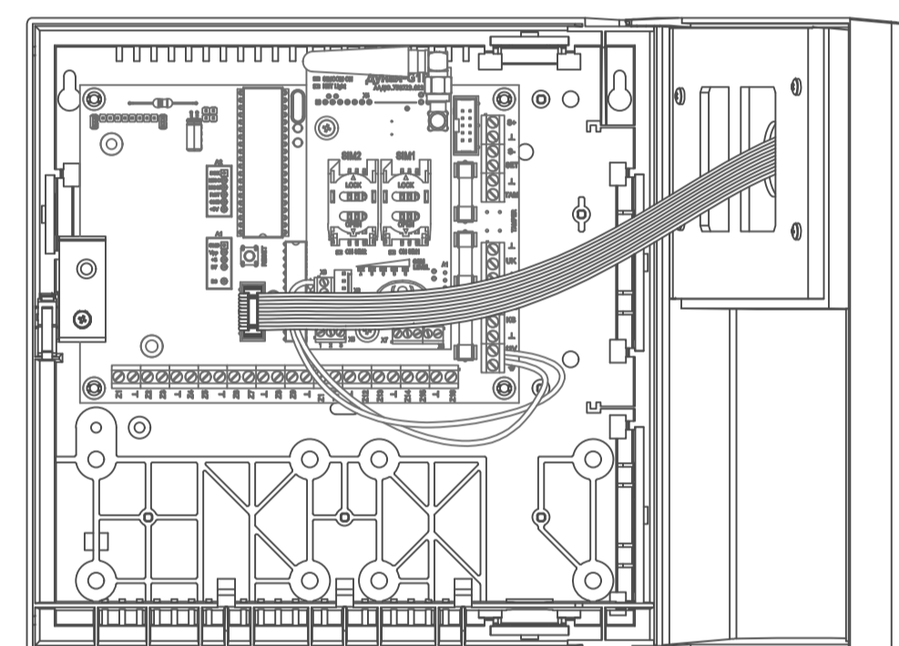
ПККОП "Данна-16/32" + Модуль "Данна-С1С" (крышка открыта)
