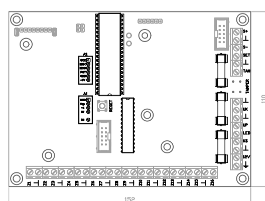
Системная плата "Данна-С1С6"
